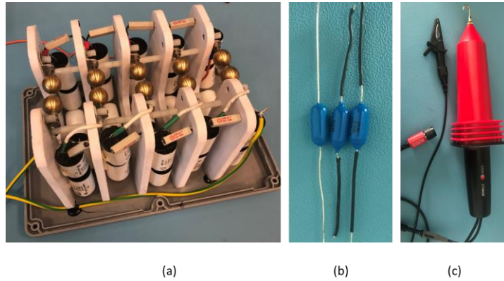
Şekil 2. (a) Kompakt Marx üretici, (b) Yük dirençleri ve (c) Cal Test CT4028 gerilim alması
