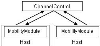
Şekil 2. Hareketlilik Mimarisi.
