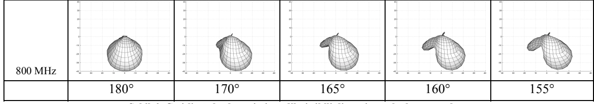
Şekil 6: Çeşitli yönlerde optimize edilmiş ikili dizgenin uzak alan ışınımları.
