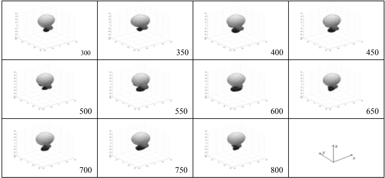
Şekil 2. Frekansa (MHz) bağı uzak alan ışıma grafikleri.
