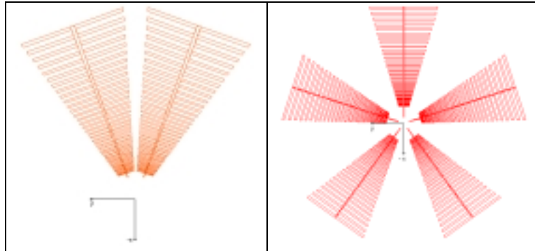
Şekil 5.a. İki log-periyodik anten dizgesi. Şekil 5.b. Beşli log-periyodik anten dizgesi.
