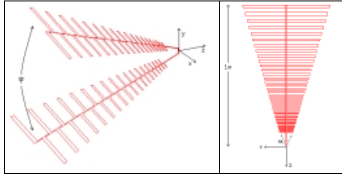
Şekil 1. Log-periyodik anten tasarımı.
