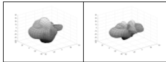
Şekil 7. Beşli dizge, uzak alan ışınımları.
